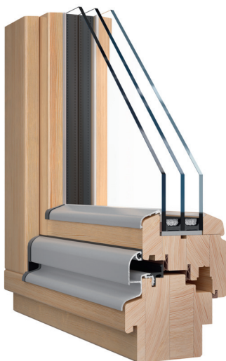
▲ Fot. 4 – Przekroje poprzeczne przez pionowe i poziome profile okna ELITE 92.
